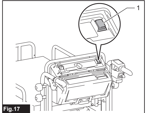
► 1. Commutateur de déplacement vers le haut et vers le bas
